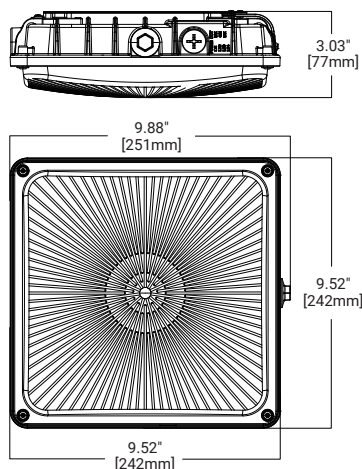
CLCS15S-PC
